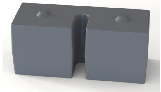
257x98x110mm 18.3kg Zwischenraum 22mm Ref. CT20 V2SN
