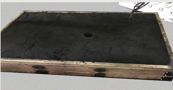
SCHLIESSEN DER BEIDEN HALBSANDFORMEN
