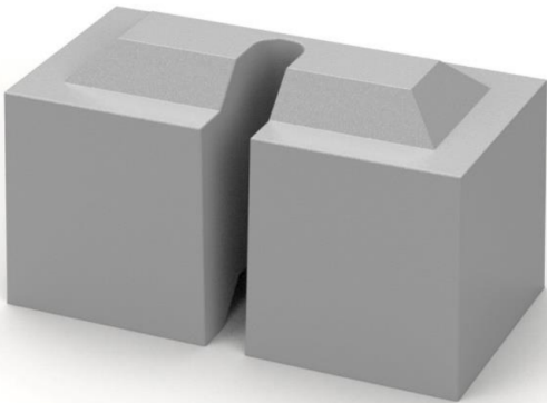
230x120x110mm 20.7kg Zwischenraum 20mm Ref. CP232 122 155
