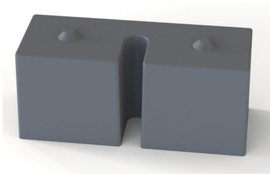
253x98x110mm 18.2kg Zwischenraum 22mm Ref. CTP20 FONTE1
